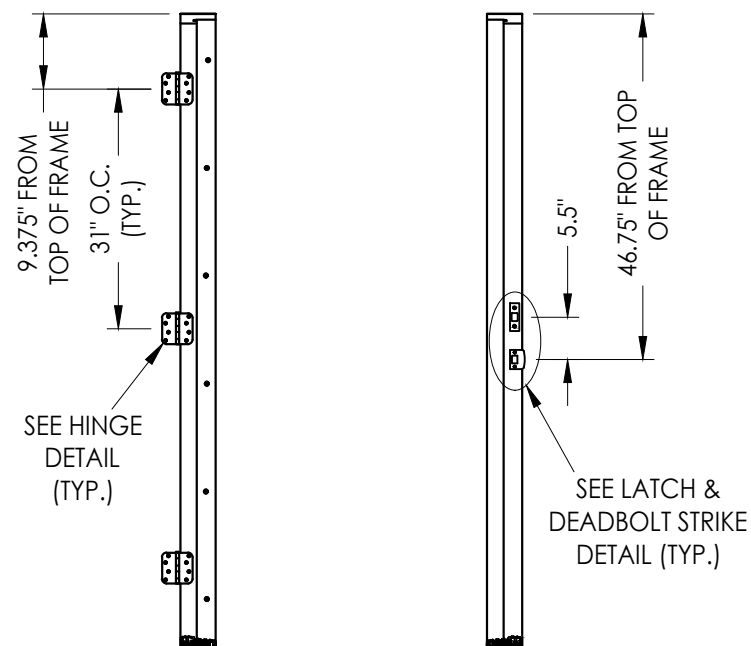
HINGE JAMB
